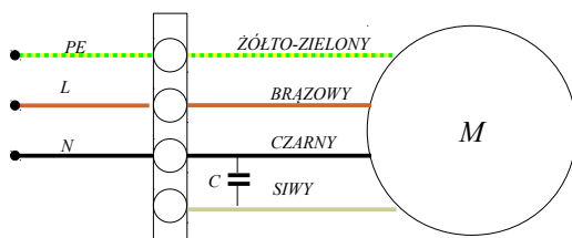
Podłączenie Silnia
