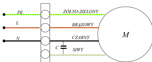
Podłączenie Silnika
