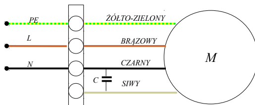
Podłączenie Silnia
